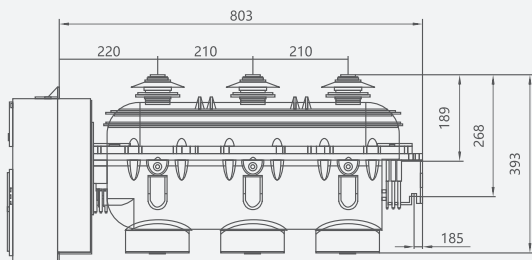
Вид сбоку
